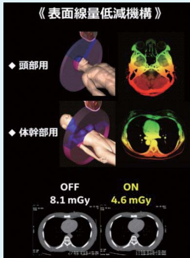
図4. 体表面被ばく線量低減機構
